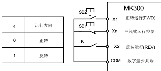
图 6-9 三线式控制模式 2
