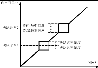
图 6-14 跳跃频率示意图
