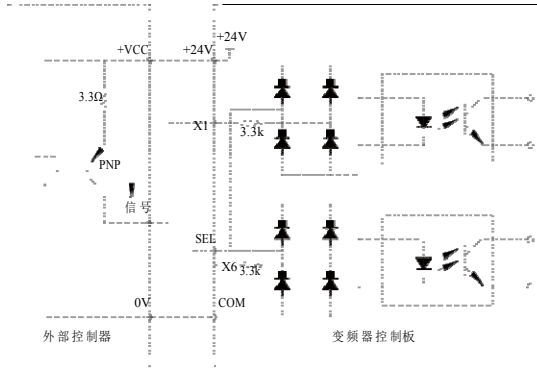
图 3-16 源型接线方式
