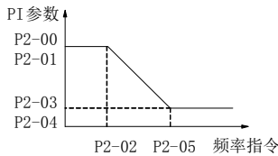
图 6-2 PI 参数示意图
