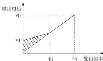
图 6-3 手动转矩提升示意图
