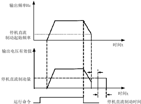
图 6-13 停机直流制动示意图
