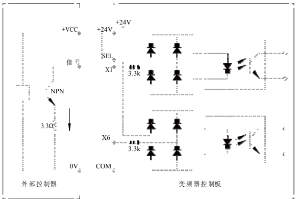
图 3-15 漏型接线方式
