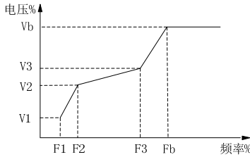
图 6-4 多点 V/F 曲线设定示意图
