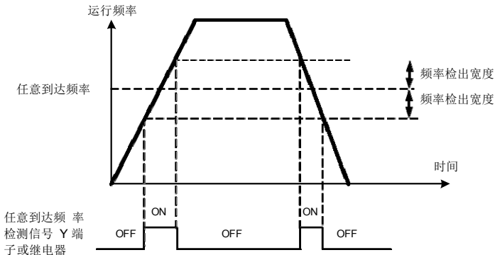
图 6-20 任意到达频率检测示意图
